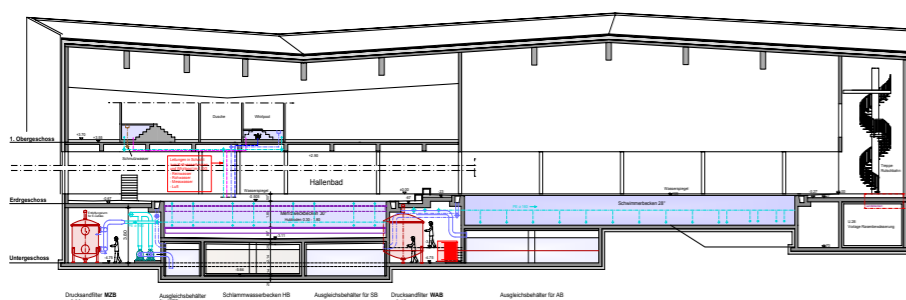
SCHNITT A - A
